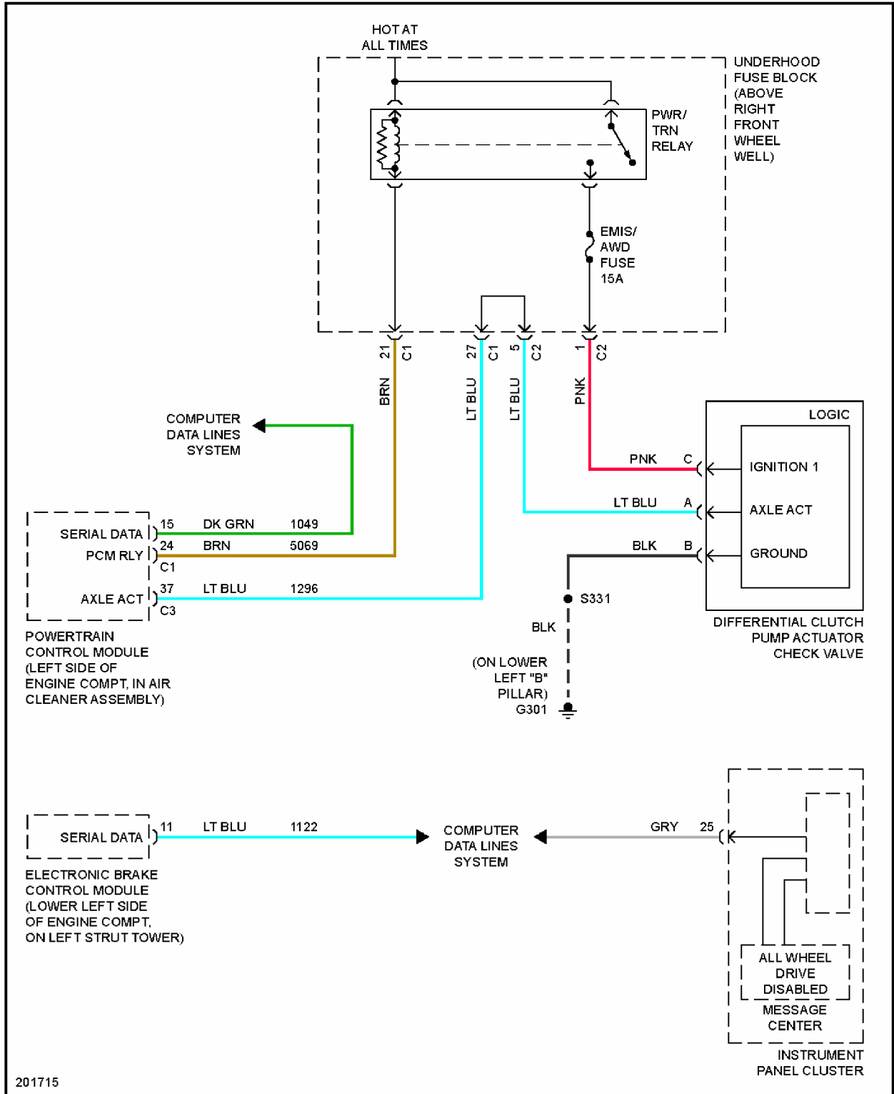
Fig. 58: AWD Circuit
