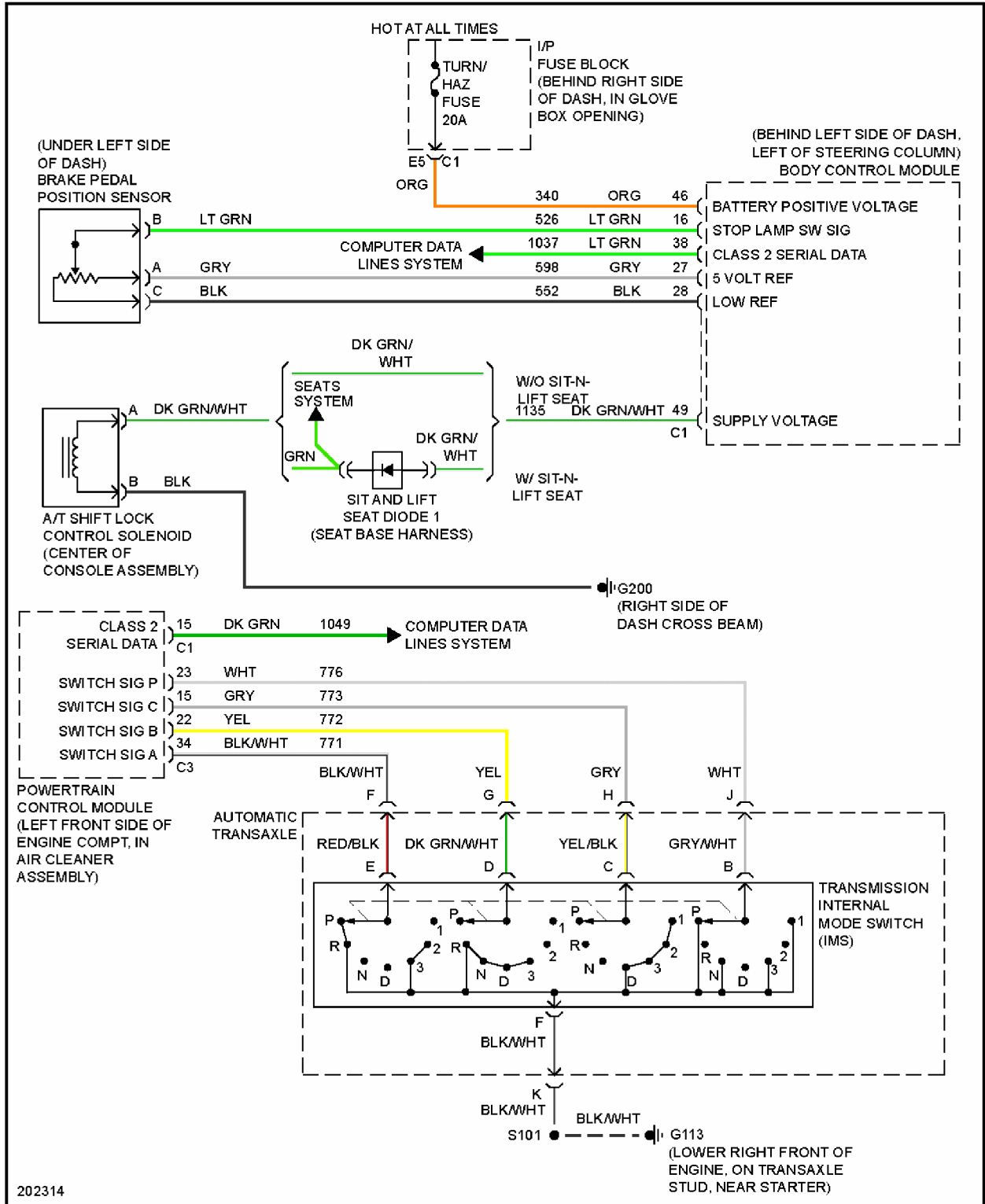
Fig. 51: Shift Interlock Circuit
